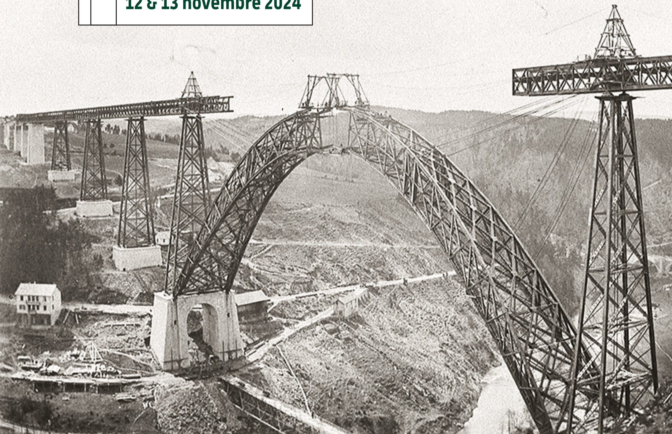
Viaduc de Garabit, Alphone Terpereau, 1884, École nationale des ponts et chaussées
